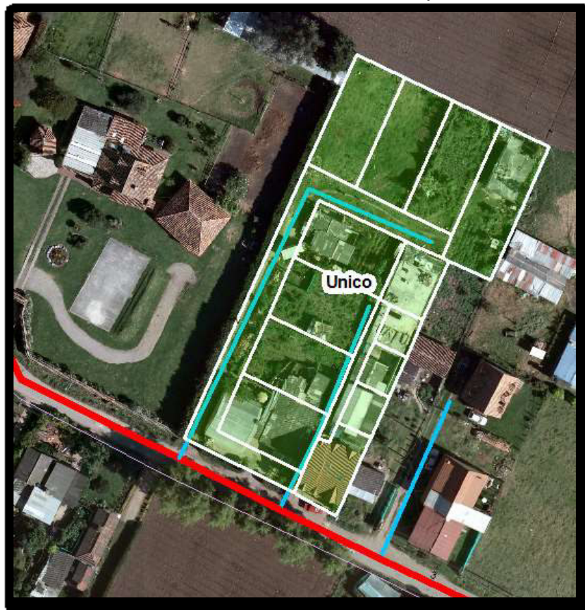
Ilustración 2. Redes existentes de acueducto zona objeto de estudio
