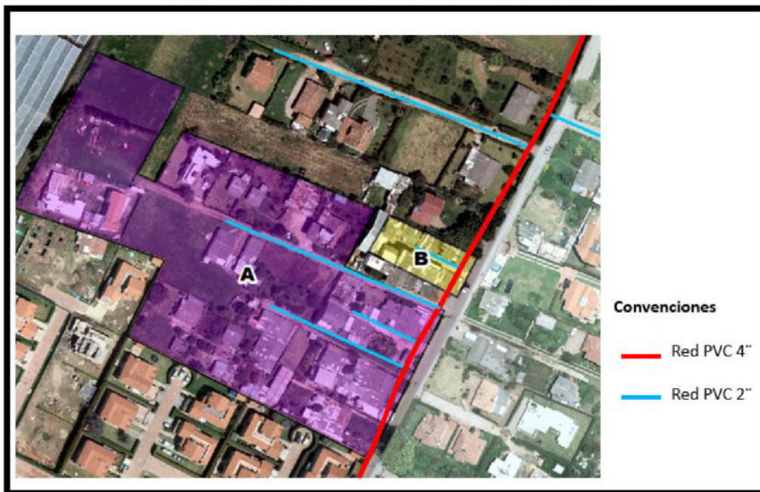
Imagen 10. Redes existentes de acueducto zona objeto de estudio
