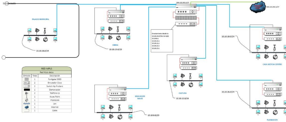
Figura 7 Arquitectura Red Servidores imagen propia
