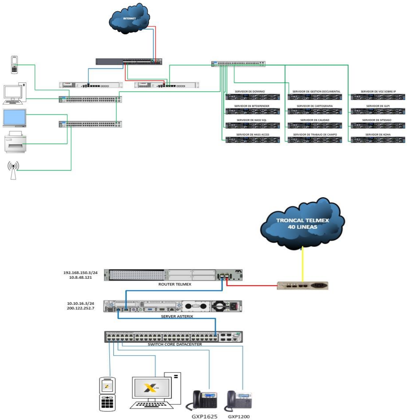
Figura 8. Arquitectura Red Telefonía imagen propia
