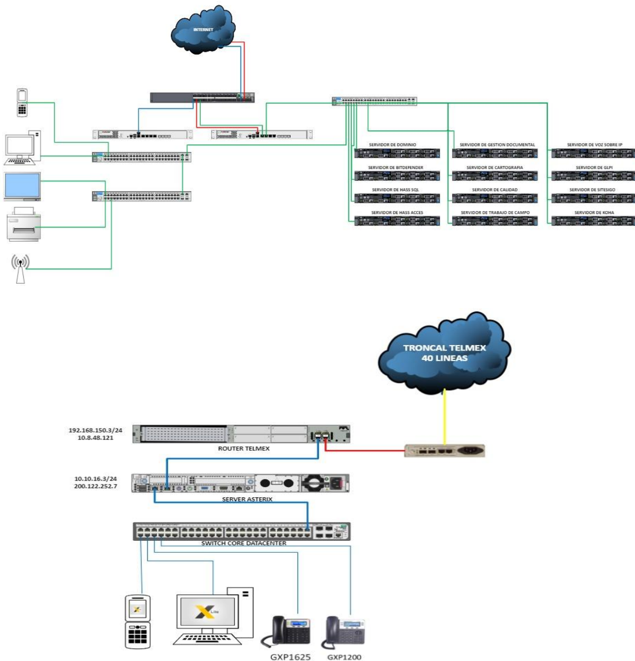
Figura 8. Arquitectura Red Telefonía imagen propia
