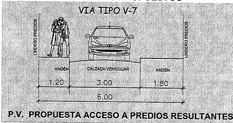
Ilustración 35: Perfil vial propuesto SERVIDUMBRE PUBLICA
