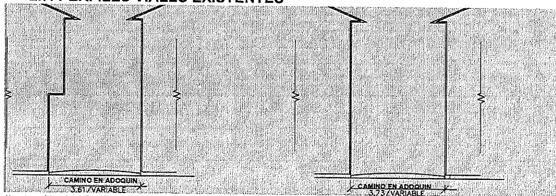
Ilustración 34: Perfil vial existente
