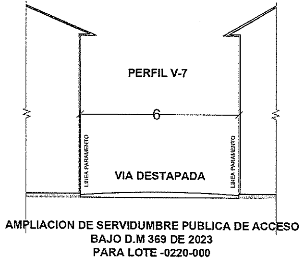
Ilustración 10: Perfil vial propuesto SERVIDUMBRE PUBLICA
