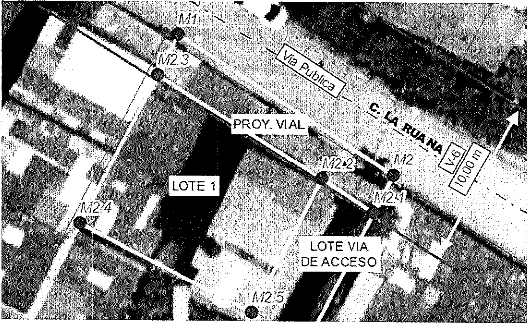
Perfil vial proyectado para la zona
